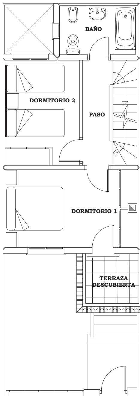
PLANTA ALTA
